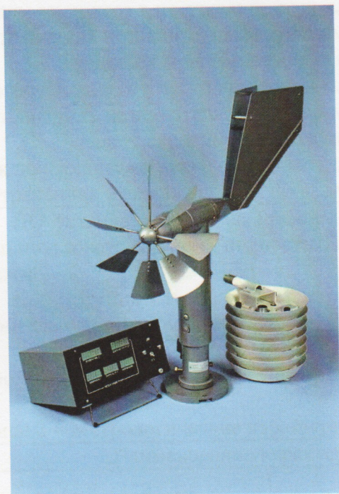
Рисунок 1 Стационарный вариант М-49М
